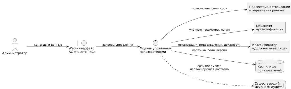
Рисунок 5 – Логическая схема интеграционных взаимодействий
