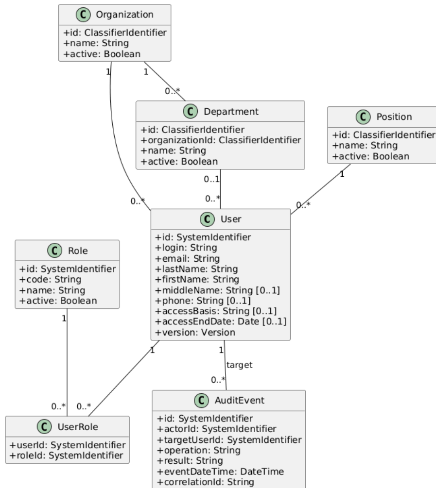
Рисунок 2 – Упрощённая логическая модель данных
