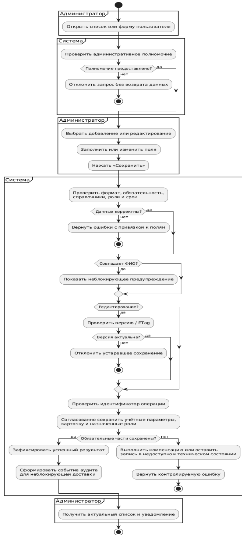
Рисунок 4 – Бизнес-процесс управления пользователем
