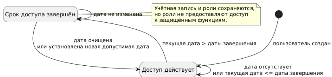
Рисунок 3 – Статусная модель срока доступа
